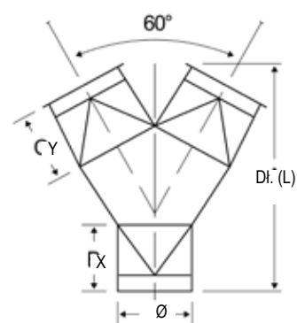
Ręczny zawór rozdzielczy RGSL / automatyczny zawór rozdzielczy RGLB
