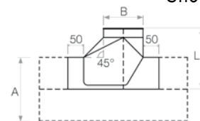
Wcinka Quick-Fit typu „Boot Shoe”
