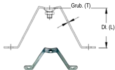
Ø 80 – 500
