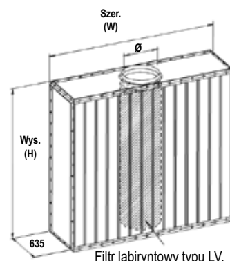
Filtr labiryntowy typu LV.
