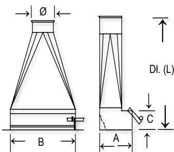
Wentylacja przypodłogowa
