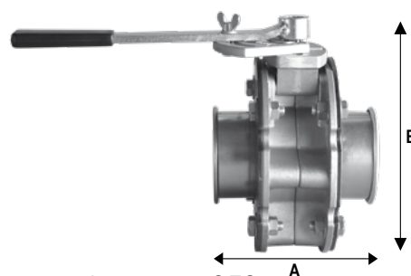
Przepustnica ręczna QFS
