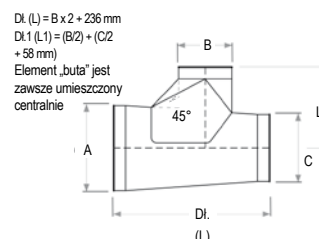
Wcinka Quick-Fit typu „Boot Shoe”
