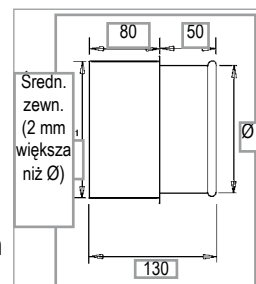
Adapter poszerzony do maszyn QFS
