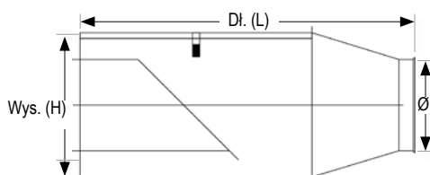
Zawór klapowy zwrotny QF
