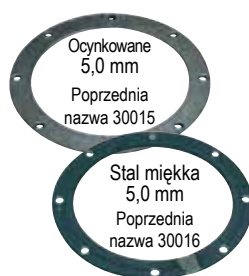
Inna poprzednia nazwa: kołnierz Nordfab
