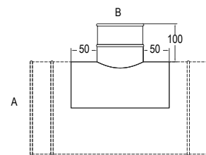
Wcinka Quick-Fit 90°
