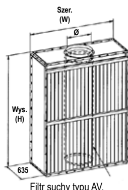
Filtr suchy typu AV.
