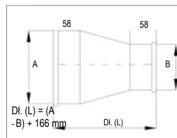
Redukcja QFS
