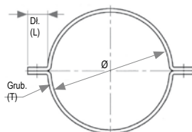
Dwuczęściowa obejma KVDA
