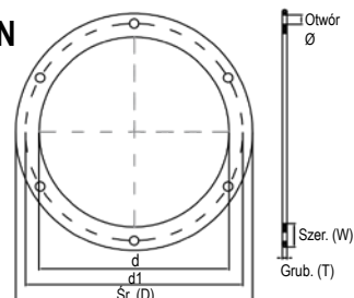
Kołnierze FLN
