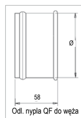
Adapter do przewodów elastycznych QF
