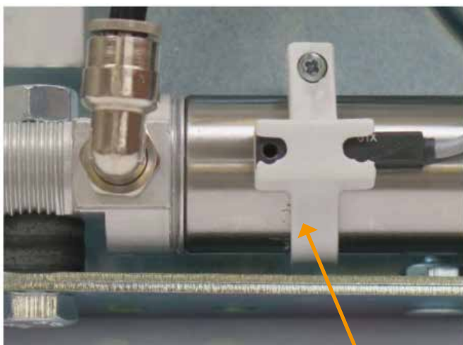
Kontaktron zamocowany na cylindrze.
