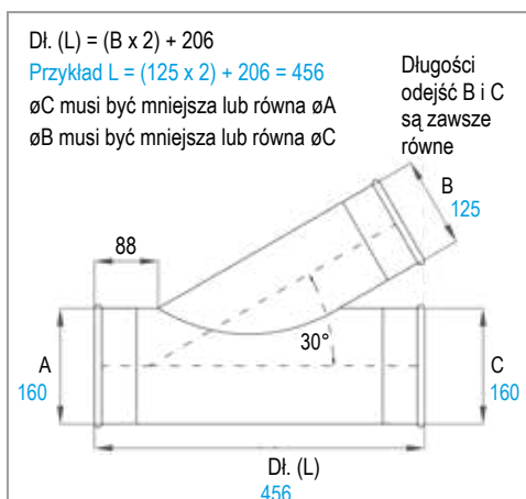
Rozgałęzienie standardowe Quick-Fit
