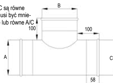
Trójnik Quick-Fit
