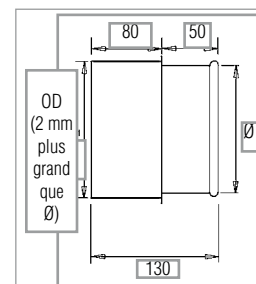
Adaptateur de machine étendu QFS
