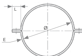
Sangle fendue KVDA
