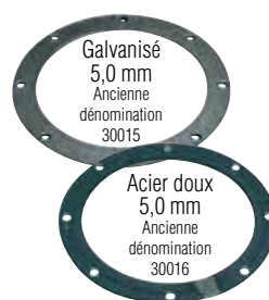
Aussi anciennement appelée bride Nordfab
