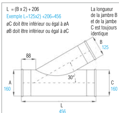
Dérivation standard Quick-Fit
