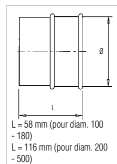
Adaptateur de ventilation QF
