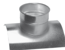
Piquage Quick-Fit à 90°
