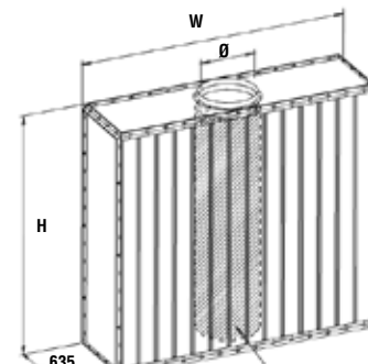
Filtre à labyrinthe de type LV.
