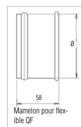
Adaptateur de tuyau QF
