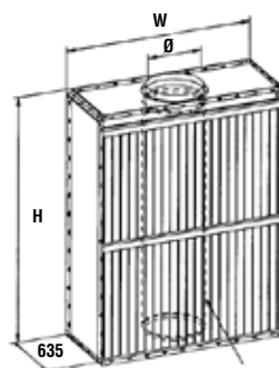
Filtre sec de type AV.
