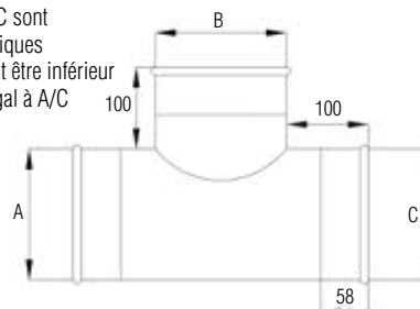
Raccord en T Quick-Fit
