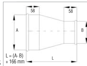
Réducteur QFS
