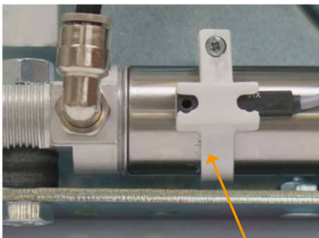
Relais Reed fixé sur le cylindre.
