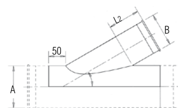
Piquage Quick-Fit à 30°
